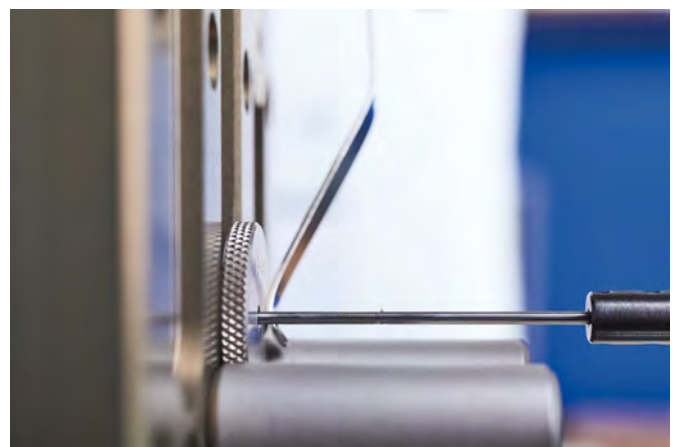
Messverfahren bei einem Gewinding
